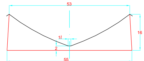
TRANSVERSAL SECTION "B" SECCION TRANSVERSAL "B"
